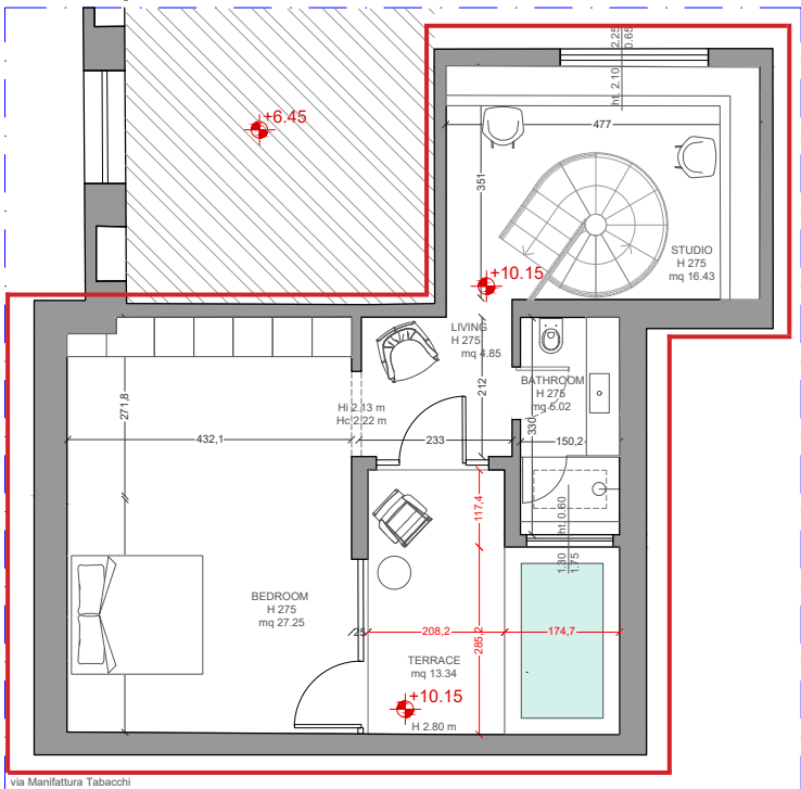
PIANTA PIANO AMMEZZATO +1 STATO DI PROGETTO
