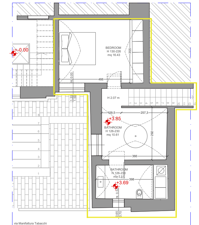
PIANTA PIANO AMMEZZATO -1 STATO DI PROGETTO
