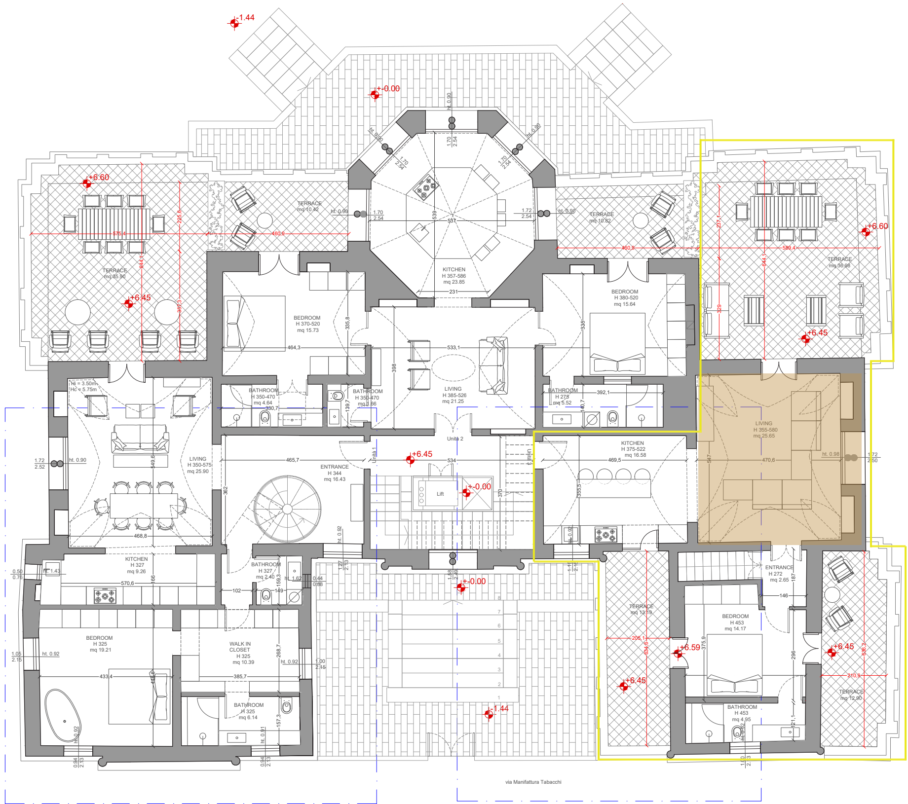
PIANTA PIANO 1 STATO DI PROGETTO
