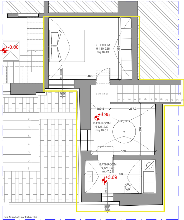
PIANTA PIANO AMMEZZATO -1 STATO DI PROGETTO
