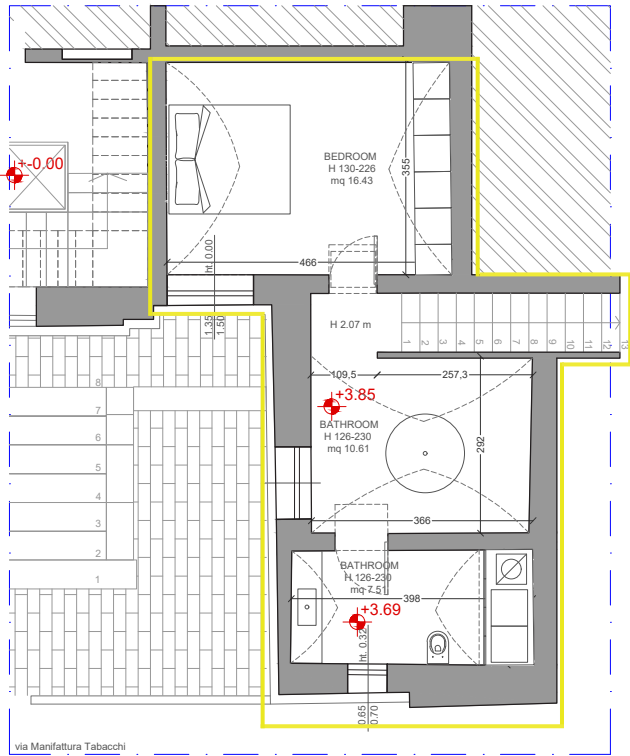
PIANTA PIANO AMMEZZATO -1 STATO DI PROGETTO
